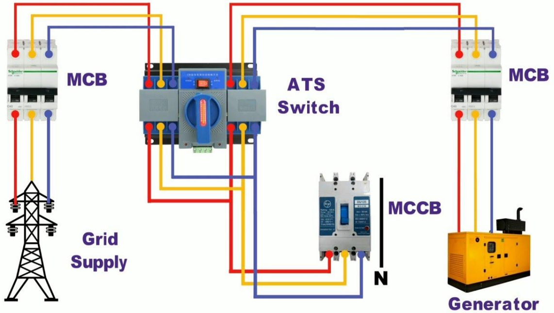
প্রি ফেজ অটোমেটিক ট্রান্সফার সুইচ
