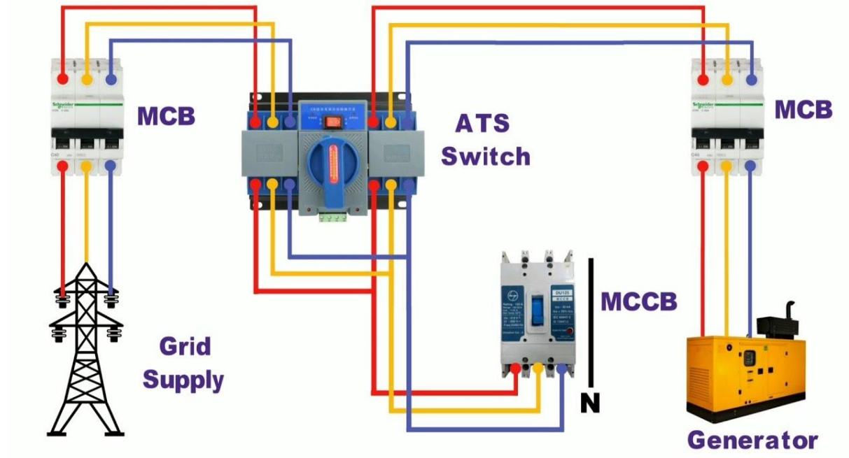
প্রি ফেজ অটোমেটিক ট্রান্সফার সুইচ
